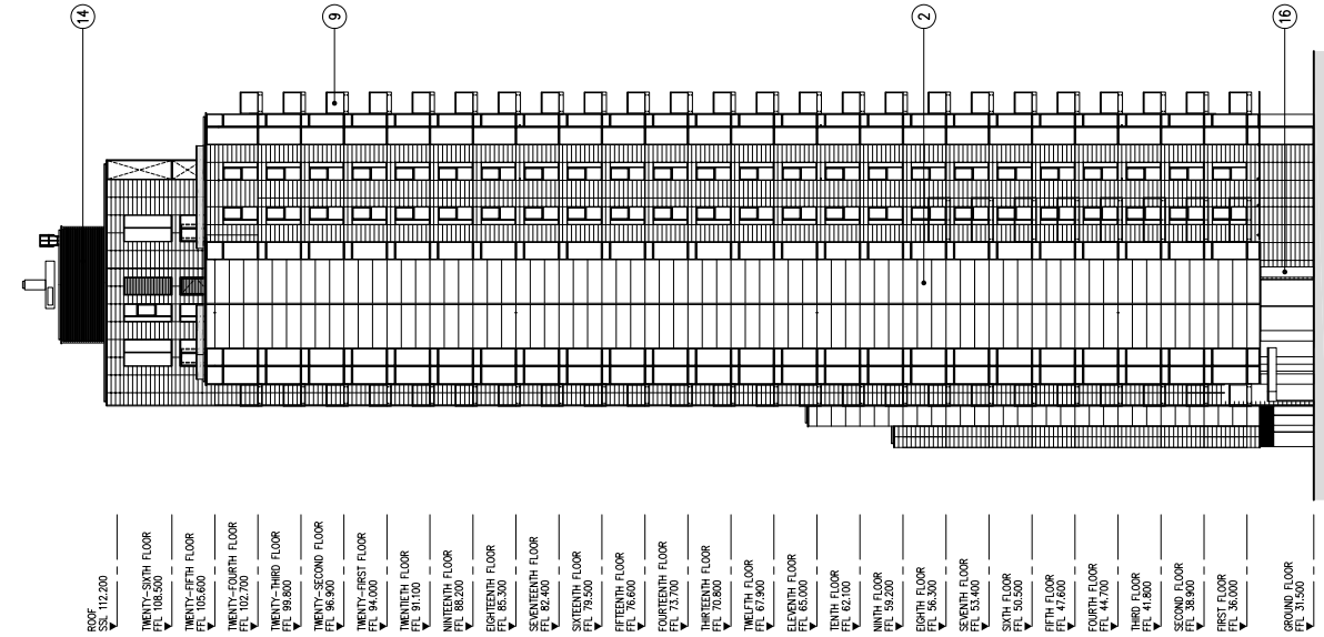
01 NORTH ELEVATION SCALE: 1:200 (A1)
