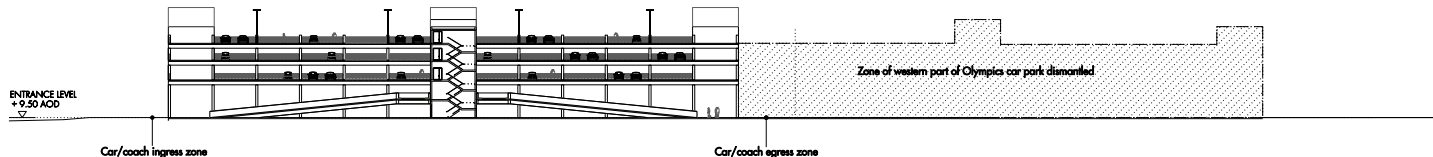
01 SECTION 01
